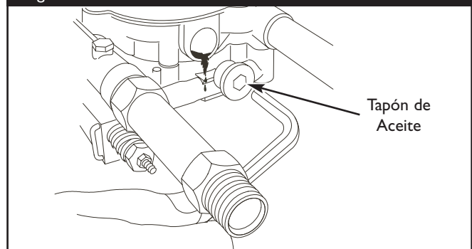
Figura 42 - Cambio del Aceite de la Bomba
